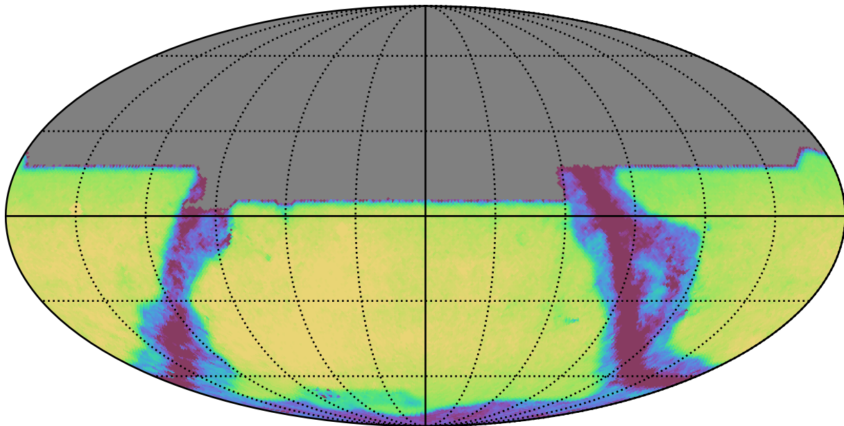
smc_lmc_v3.3_10yrs All sky y band: Exgal_CoaddM5
