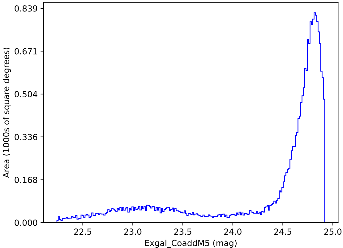
smc_lmc_v3.3_10yrs All sky y band: Exgal_CoaddM5
