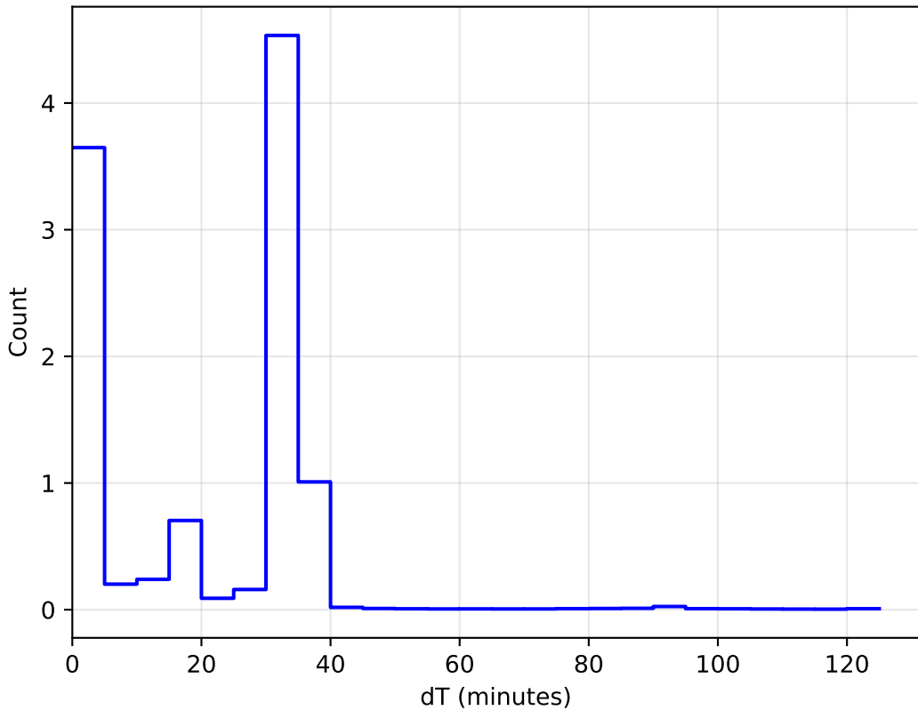
1e6 smc_lmc_v3.3_10yrs WFD: DeltaT Histogram
