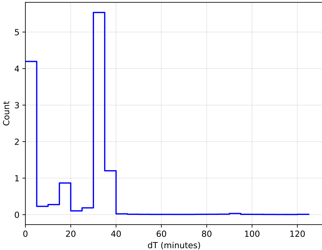
1e6 smc_lmc_v3.3_10yrs All sky: DeltaT Histogram
