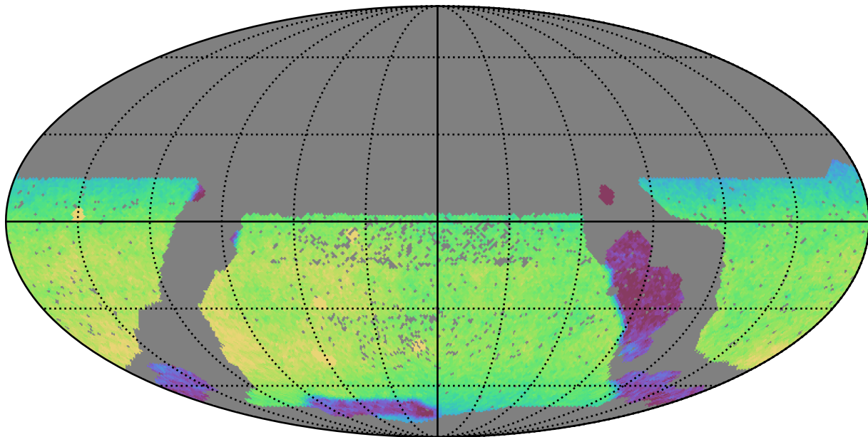
smc_lmc_v3.3_10yrs WFD y band: CoaddM5
