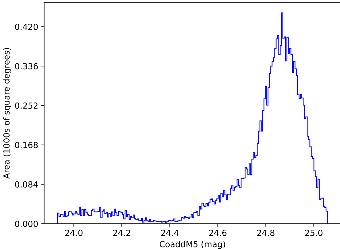
smc_lmc_v3.3_10yrs WFD y band: CoaddM5
