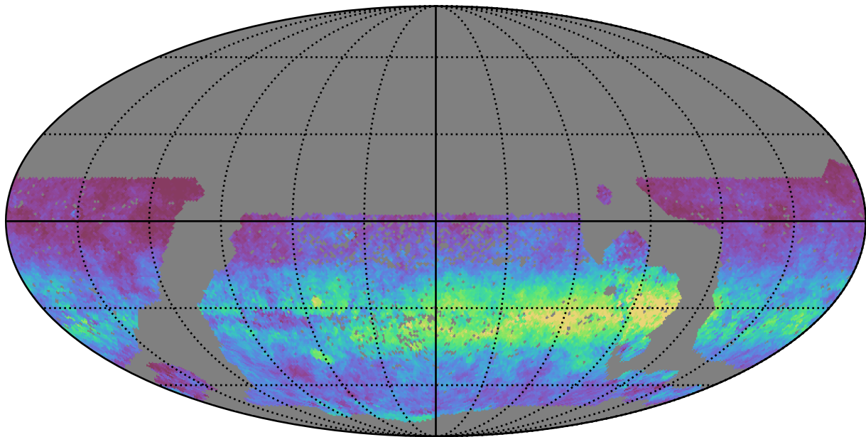
smc_lmc_v3.3_10yrs WFD y band: AngleRms rotSkyPos
