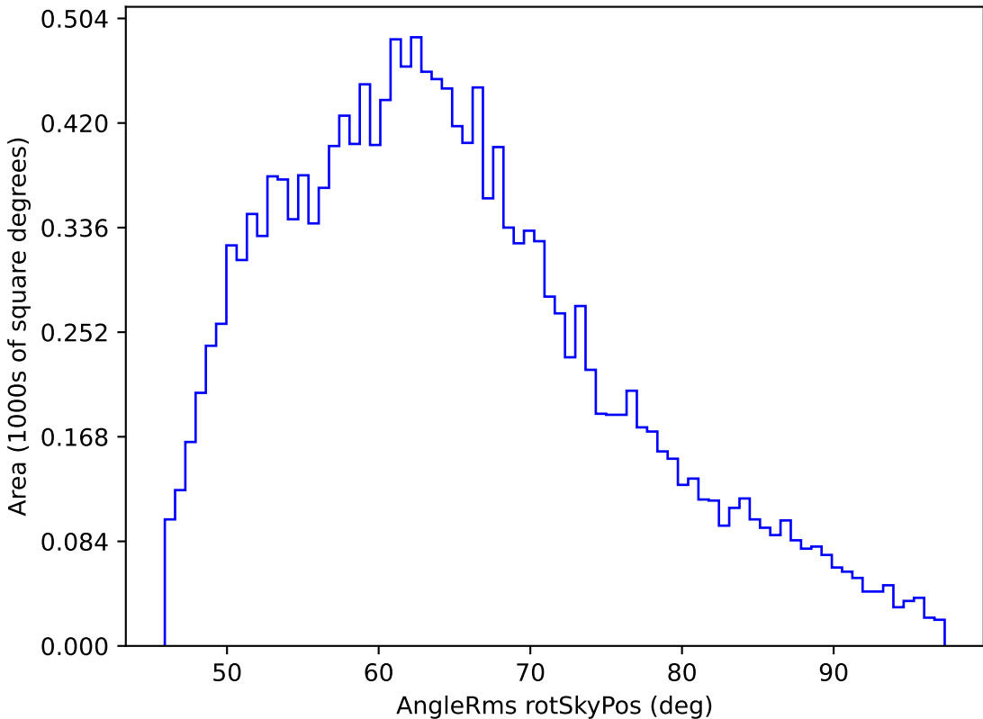
smc_lmc_v3.3_10yrs WFD y band: AngleRms rotSkyPos
