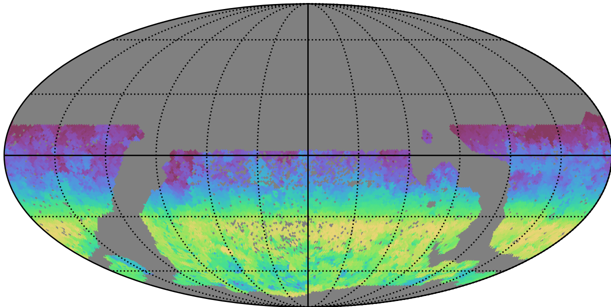
smc_lmc_v3.3_10yrs WFD z band: AngleRange rotSkyPos
