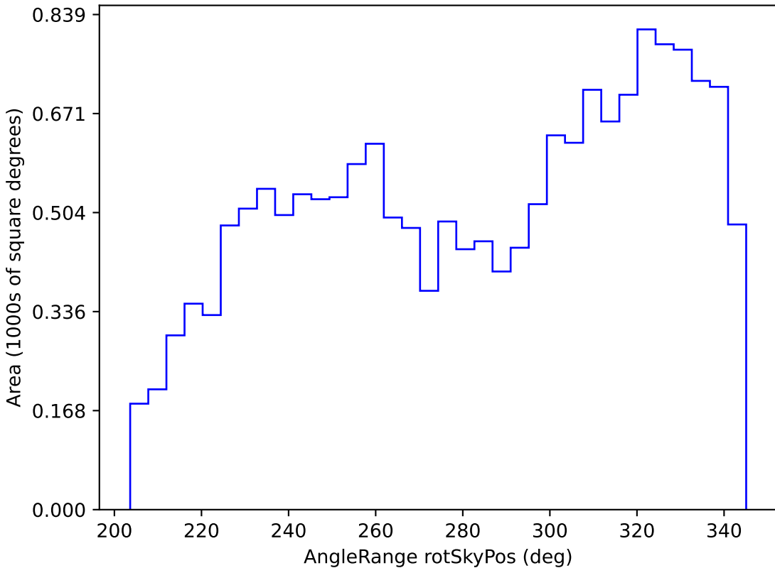
smc_lmc_v3.3_10yrs WFD z band: AngleRange rotSkyPos
