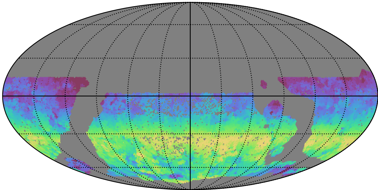
smc_lmc_v3.3_10yrs WFD y band: AngleRange rotSkyPos
