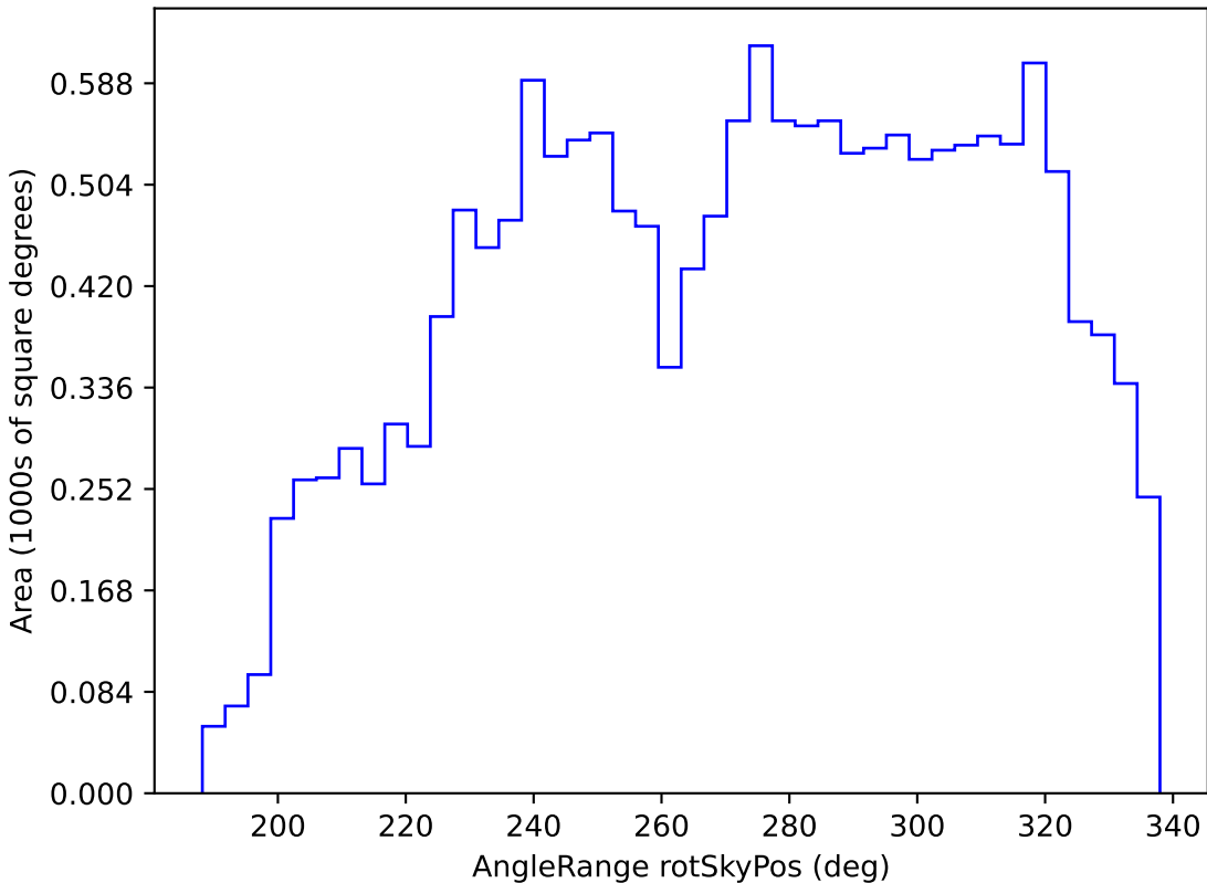
smc_lmc_v3.3_10yrs WFD y band: AngleRange rotSkyPos
