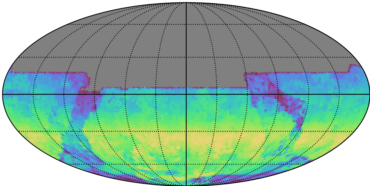
smc_lmc_v3.3_10yrs All sky y band: AngleRange rotSkyPos
