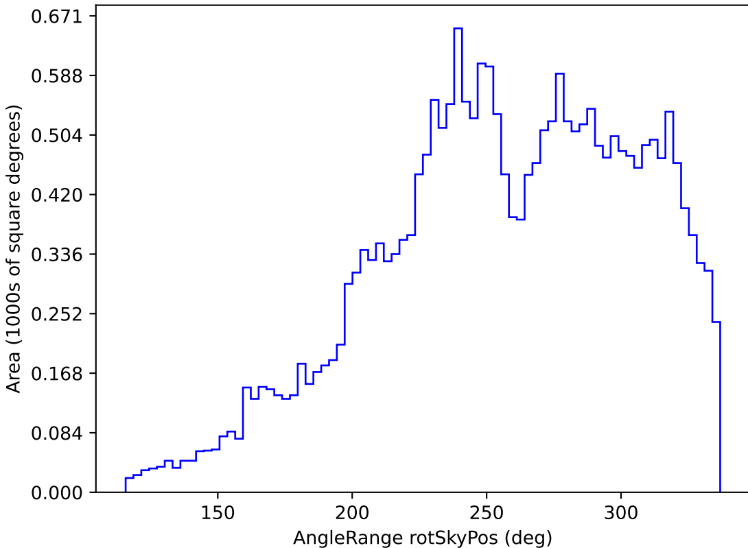
smc_lmc_v3.3_10yrs All sky y band: AngleRange rotSkyPos
