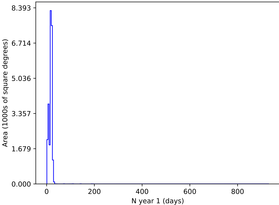
smc_lmc_v3.3_10yrs y and night < 365: N year 1
