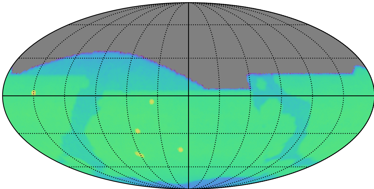
smc_lmc_v3.3_10yrs i: CoaddM5
