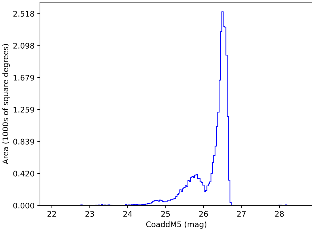
smc_lmc_v3.3_10yrs i: CoaddM5
