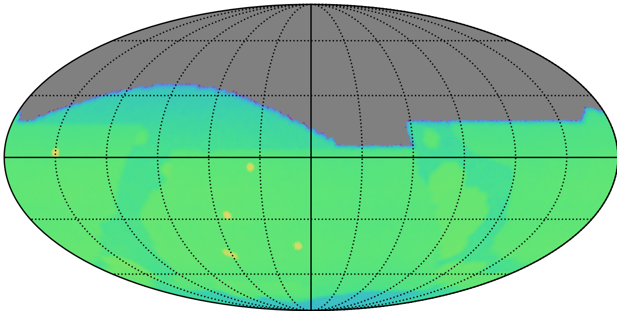
smc_lmc_v3.3_10yrs : CoaddM5
