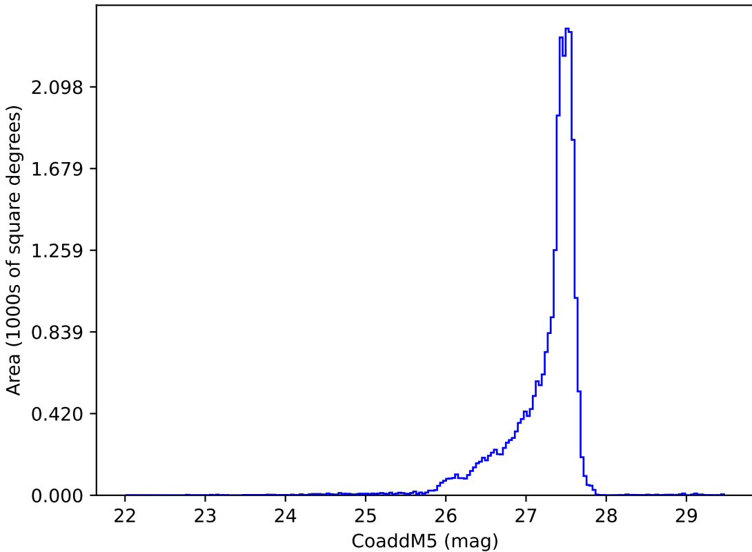
smc_lmc_v3.3_10yrs : CoaddM5
