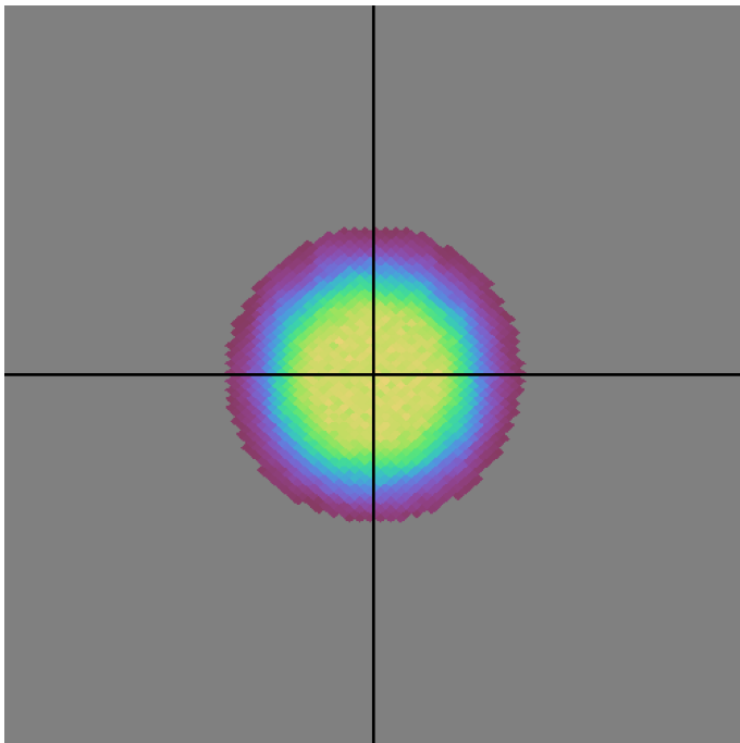
smc_lmc_v3.3_10yrs y band: DD:XMM_LSS NVisits
