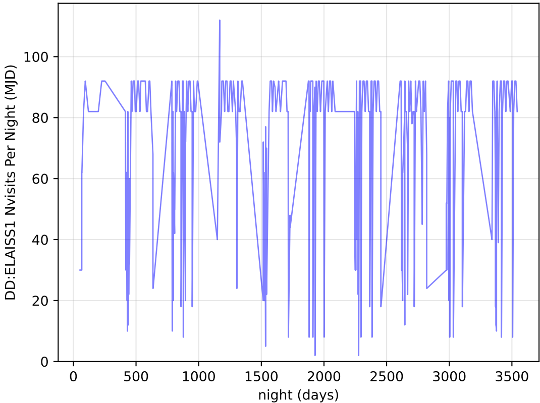
smc_lmc_v3.3_10yrs all bands: DD:ELAISS1 Nvisits Per Night
