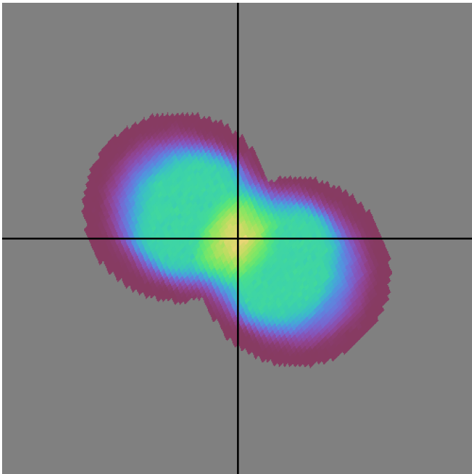
smc_lmc_v3.3_10yrs z band: DD:EDFS NVisits
