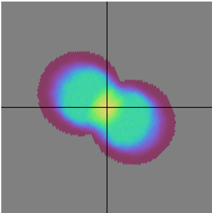
smc_lmc_v3.3_10yrs r band: DD:EDFS NVisits
