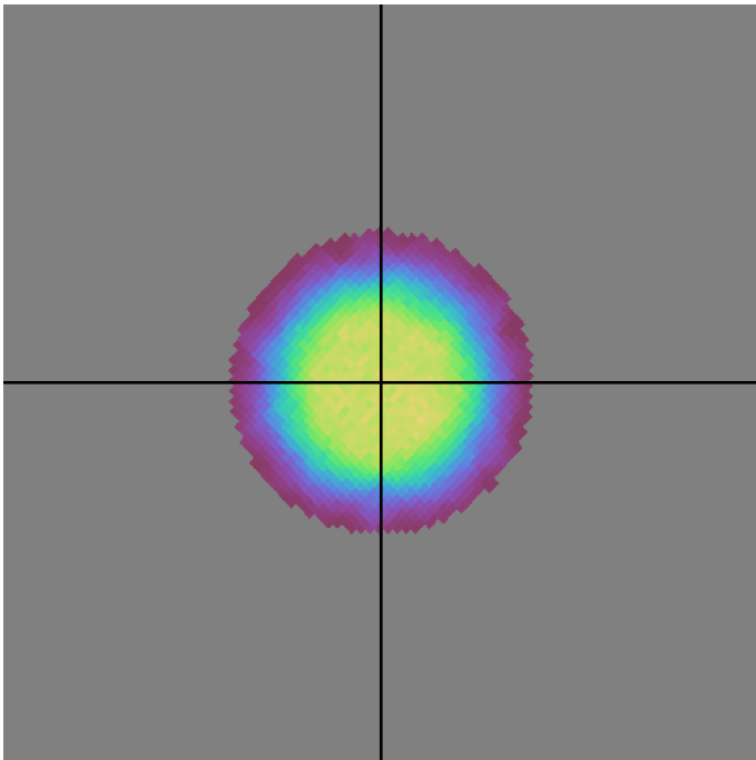
smc_lmc_v3.3_10yrs y band: DD:ECDFS NVisits
