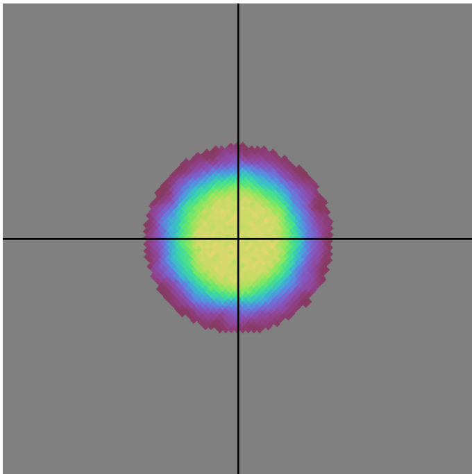
smc_lmc_v3.3_10yrs r band: DD:ECDFS NVisits
