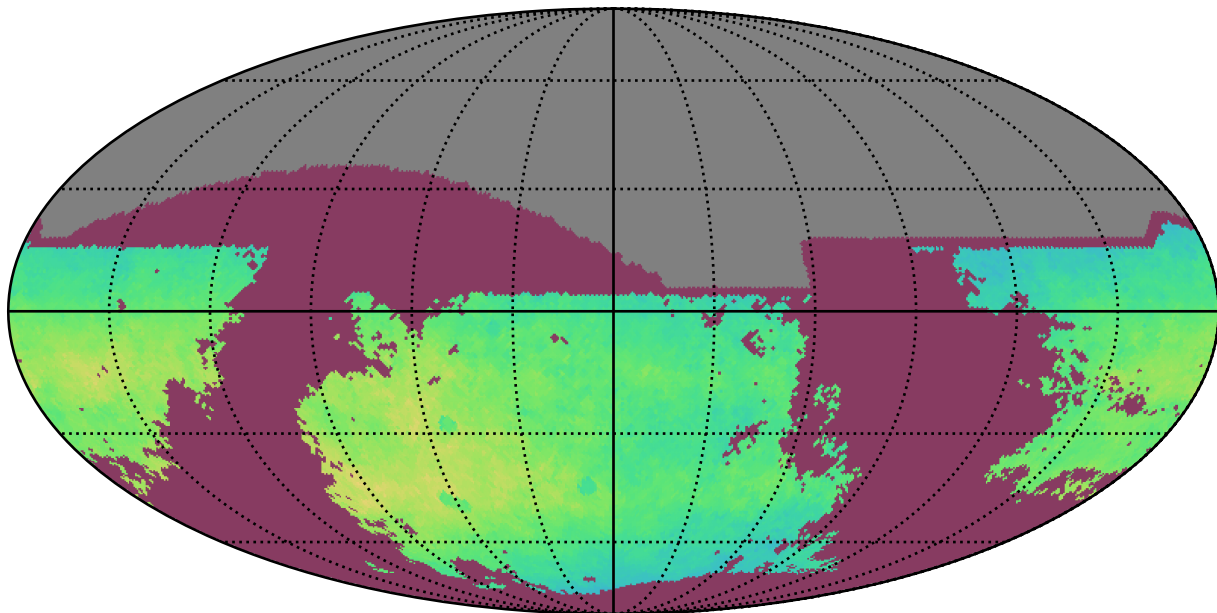
scp_reweight_v3.3_10yrs i: NgalScale
