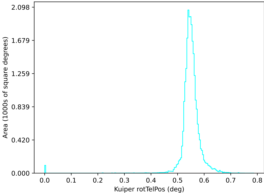
scp_reweight_v3.3_10yrs u: Kuiper rotTelPos
