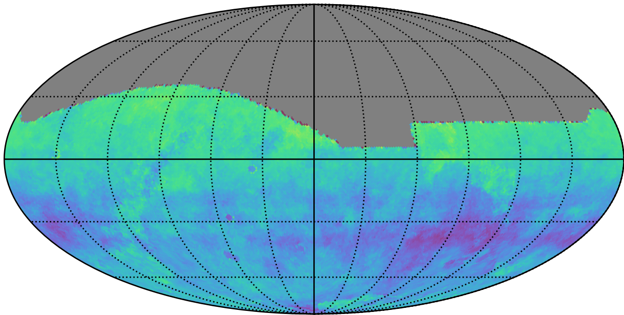
scp_reweight_v3.3_10yrs i: Kuiper rotSkyPos
