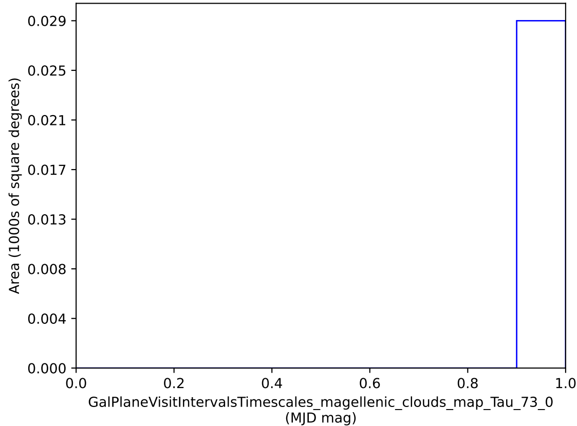
scp_reweight_v3.3_10yrs : GalPlaneVisitIntervalsTimescales_magellenic_clouds_map_Tau_73_0
