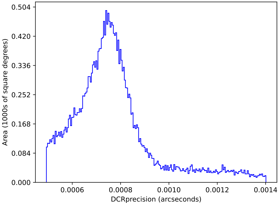
scp_reweight_v3.3_10yrs : DCRprecision
