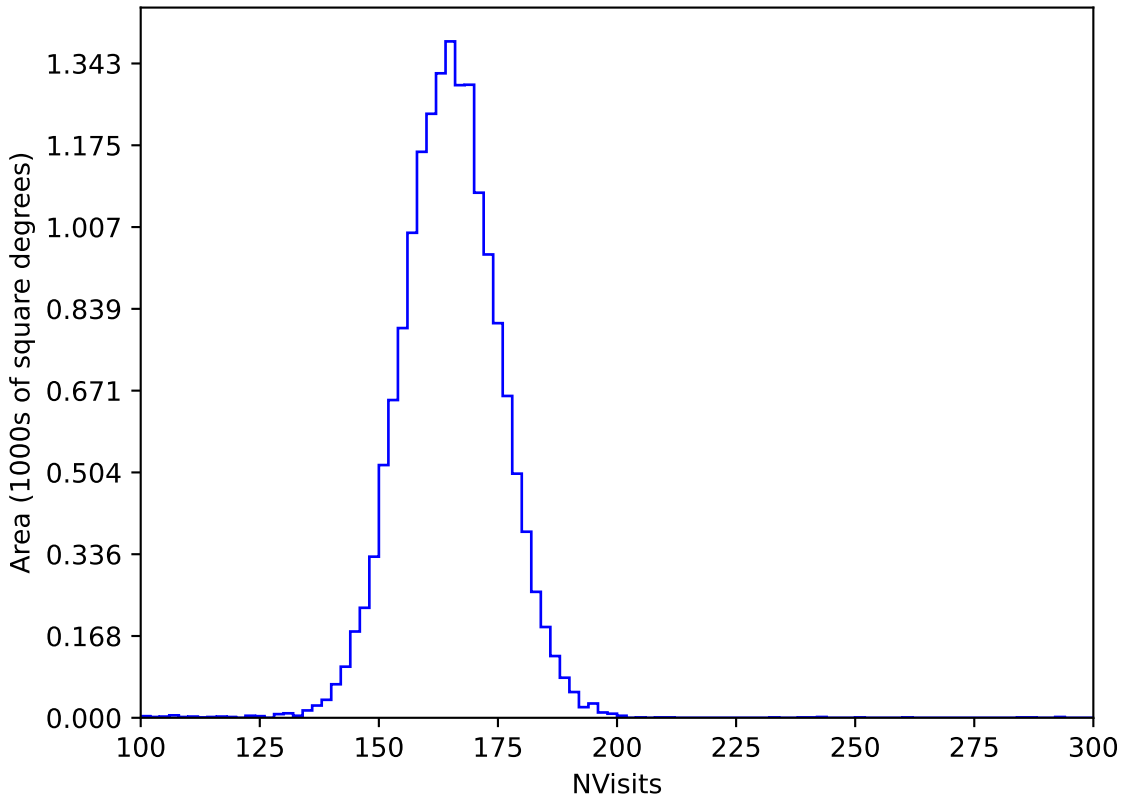
scp_reweight_v3.3_10yrs WFD y band: NVisits
