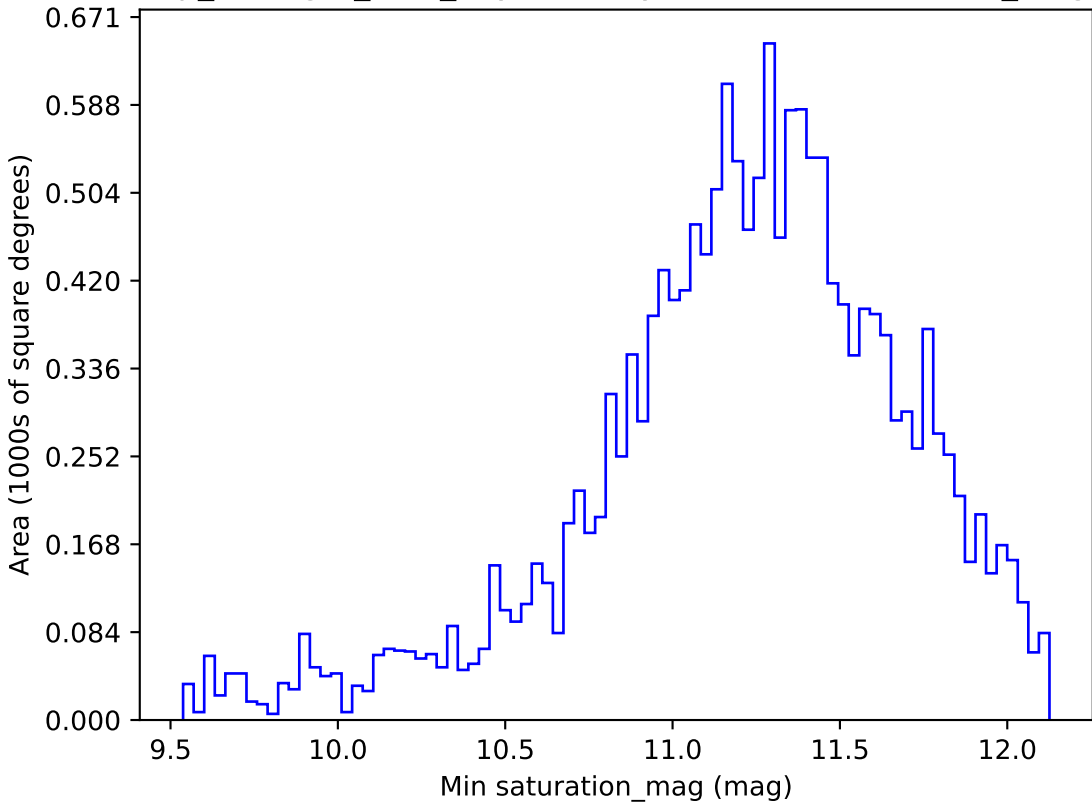
scp_reweight_v3.3_10yrs WFD y band: Min saturation_mag
