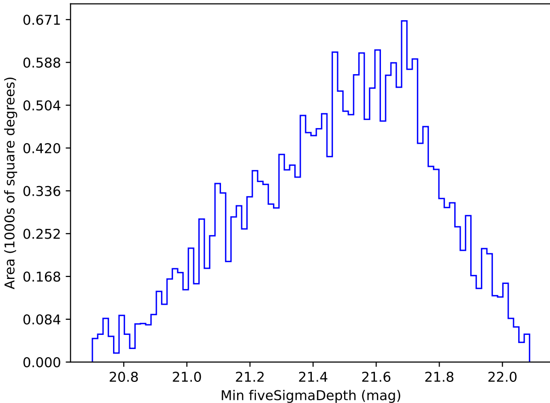
scp_reweight_v3.3_10yrs Yr 1 y band: Min fiveSigmaDepth
