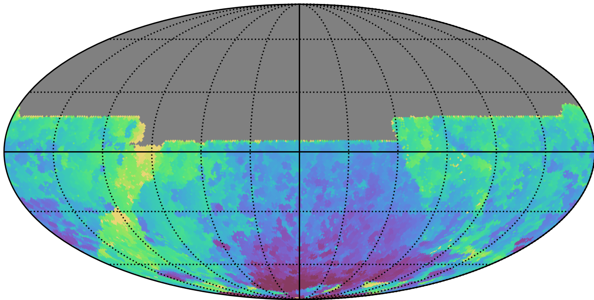
scp_reweight_v3.3_10yrs All sky y band: Min HA
