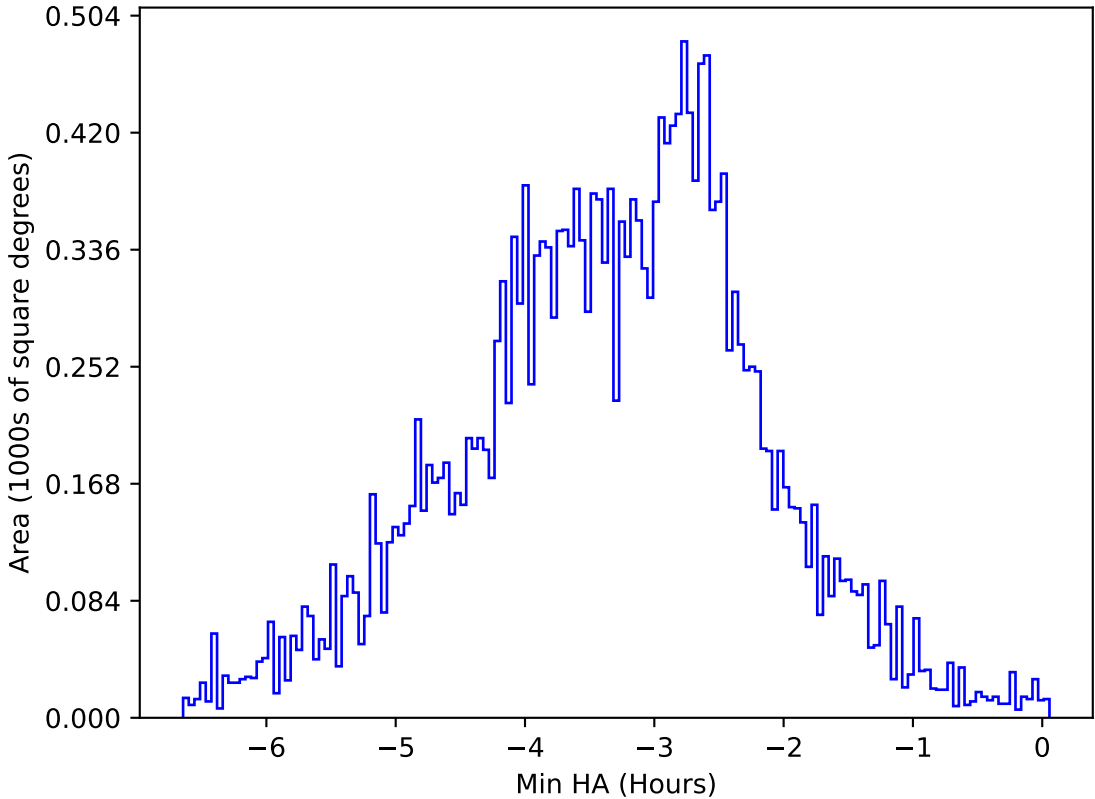
scp_reweight_v3.3_10yrs All sky y band: Min HA
