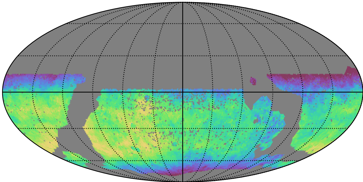
scp_reweight_v3.3_10yrs WFD y band: Median fiveSigmaDepth
