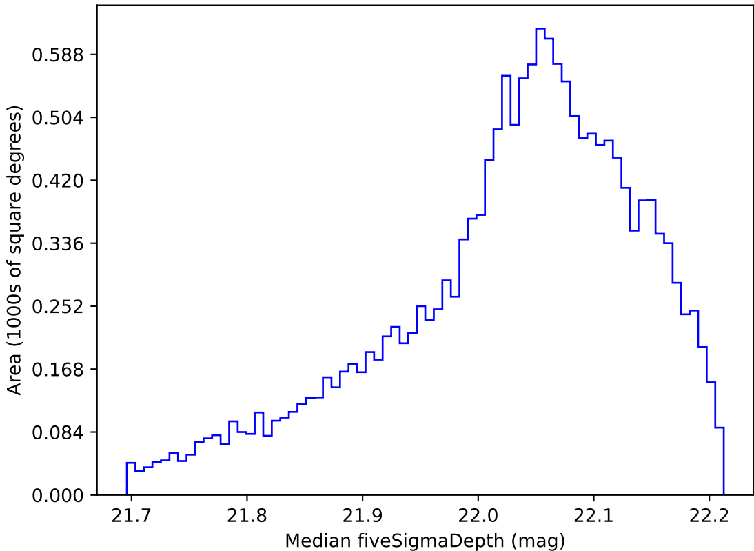
scp_reweight_v3.3_10yrs WFD y band: Median fiveSigmaDepth
