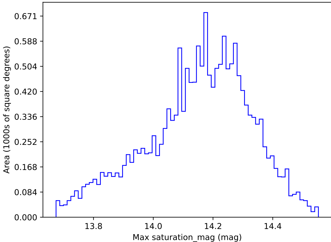
scp_reweight_v3.3_10yrs WFD y band: Max saturation_mag
