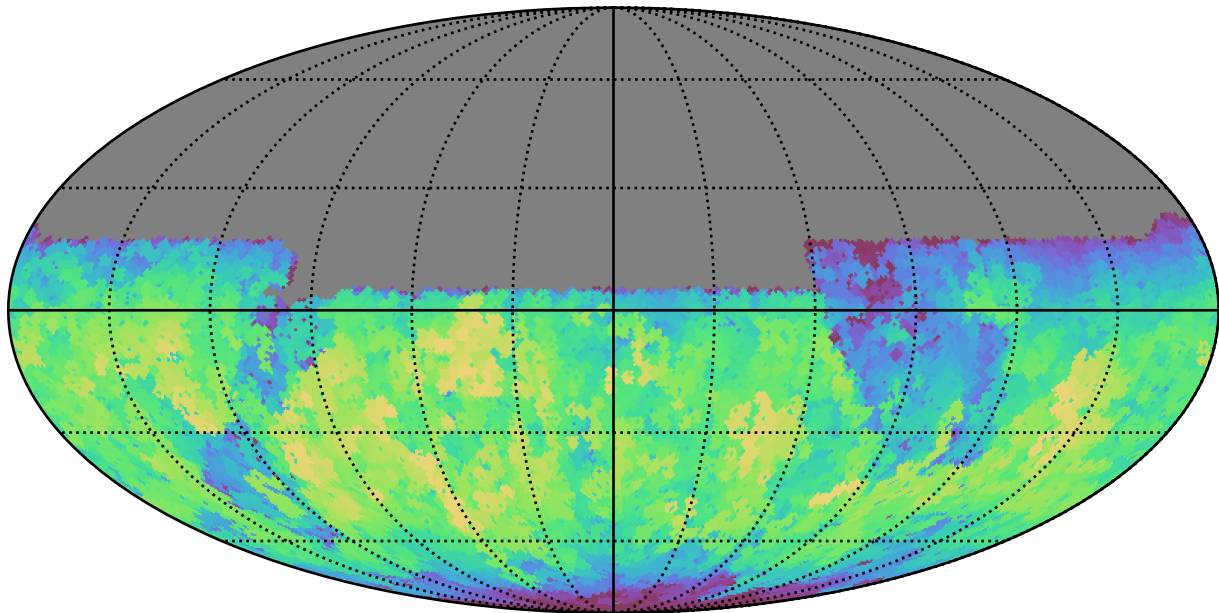
scp_reweight_v3.3_10yrs Yr 1 y band: Max fiveSigmaDepth
