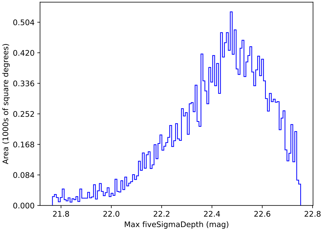
scp_reweight_v3.3_10yrs Yr 1 y band: Max fiveSigmaDepth
