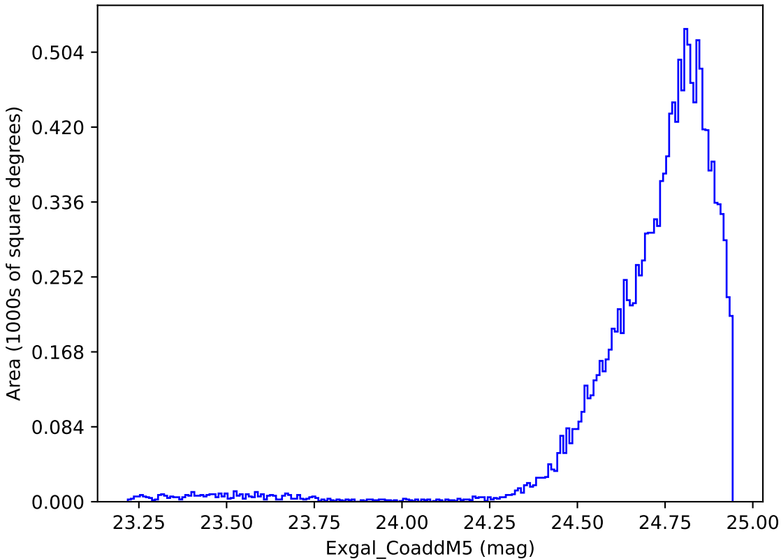
scp_reweight_v3.3_10yrs WFD y band: Exgal_CoaddM5
