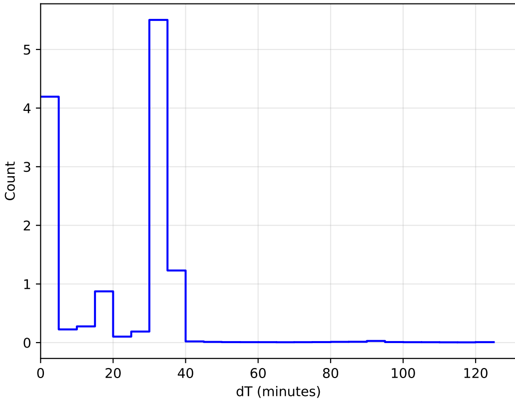
1e6 scp_reweight_v3.3_10yrs All sky: DeltaT Histogram
