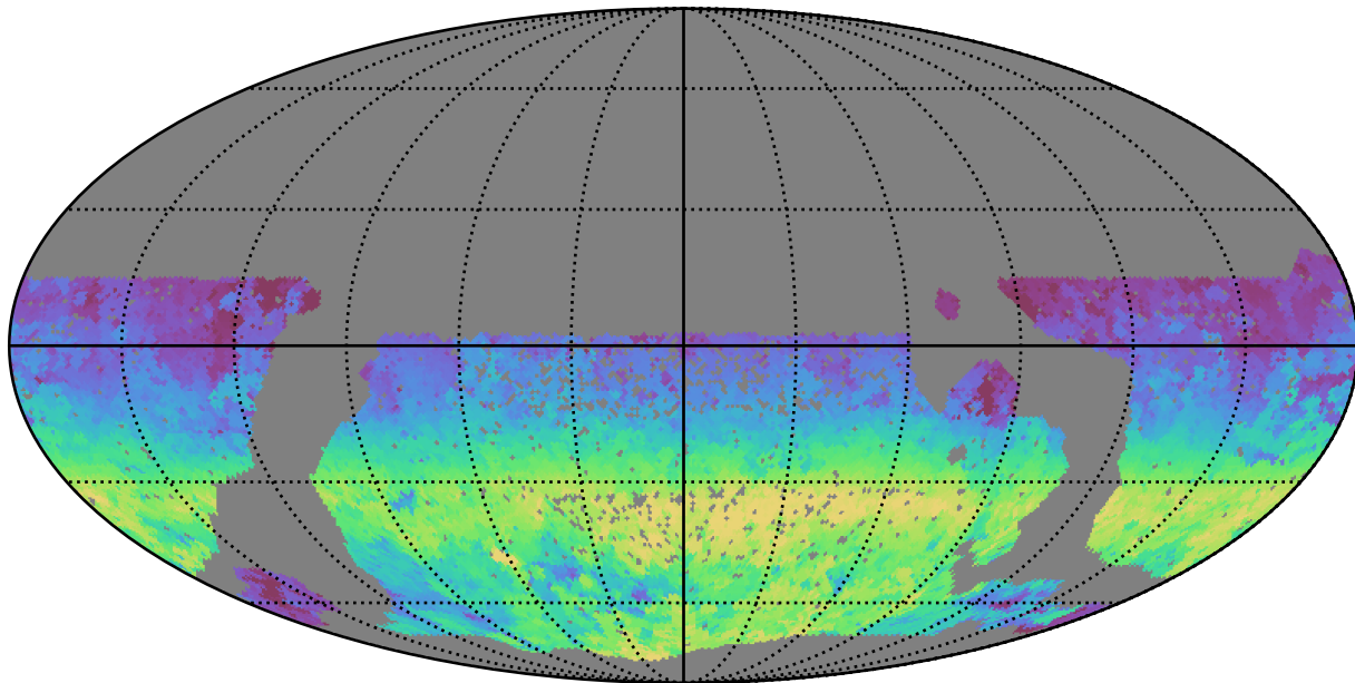
scp_reweight_v3.3_10yrs WFD y band: AngleRange rotSkyPos
