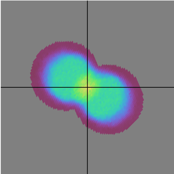
scp_reweight_v3.3_10yrs u band: DD:EDFS NVisits
