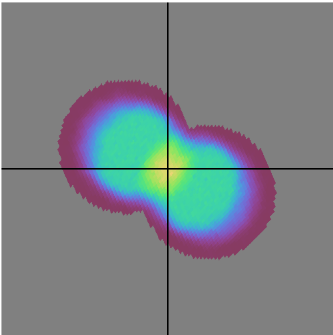
scp_reweight_v3.3_10yrs r band: DD:EDFS NVisits
