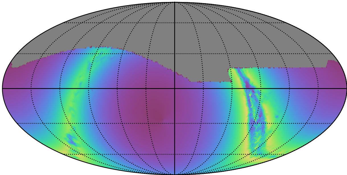
roman_v3.3_10yrs : young_stars
