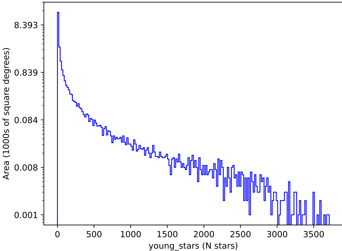
roman_v3.3_10yrs : young_stars
