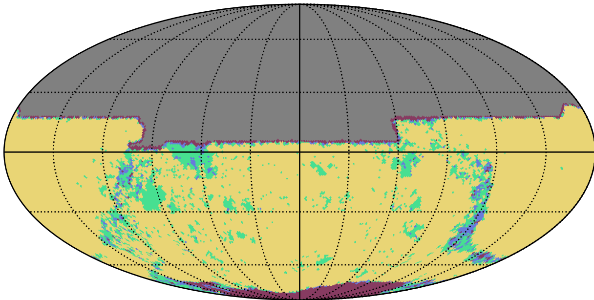
roman_v3.3_10yrs y band: YearCoverage night
