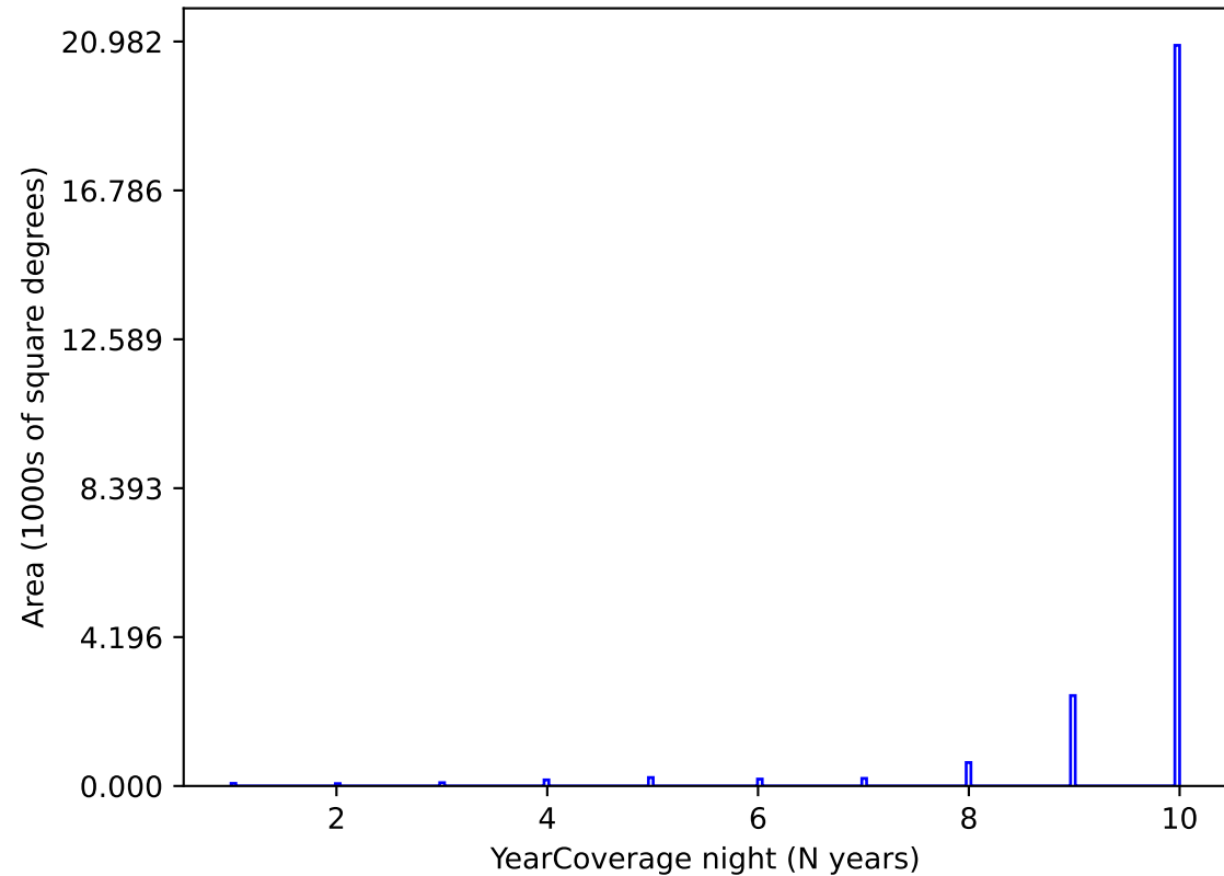
roman_v3.3_10yrs y band: YearCoverage night
