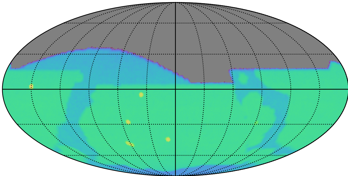
roman_v3.3_10yrs i: SurfaceBrightLimit
